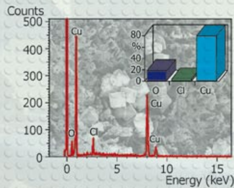
EDX-Analyse
